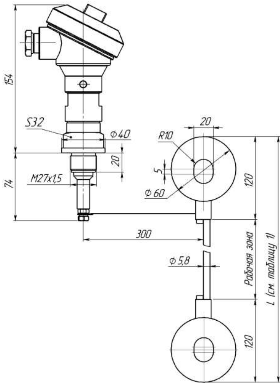
Рисунок Б.8 - ПП-095, ПП-295
