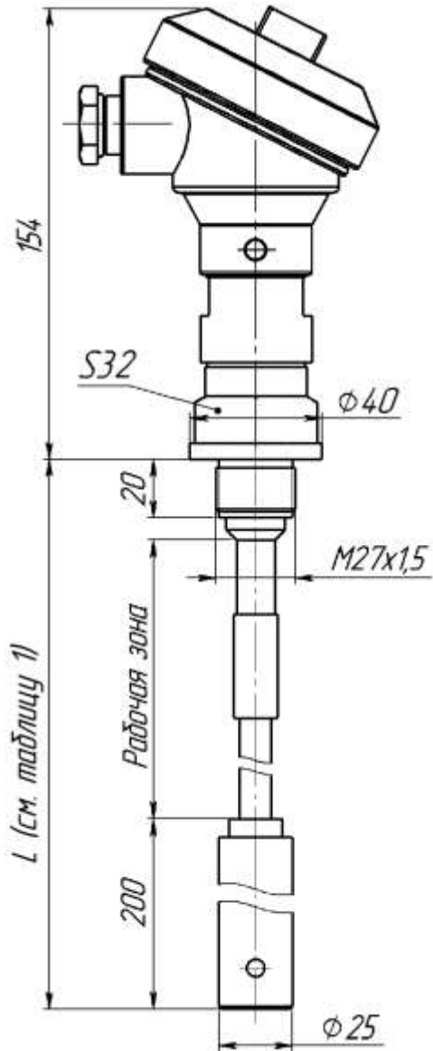
Рисунок Б.7 - ПП-094, ПП-094И, ПП-294, ПП-294И
