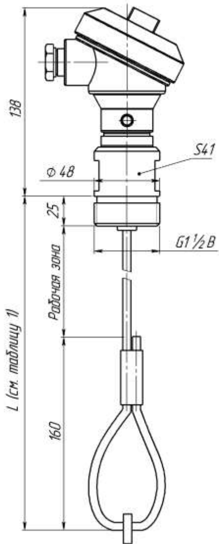
Рисунок Б.9 - ПП-092, ПП-092И, ПП-096, ПП-096И, ПП-292, ПП-292И, ПП-296, ПП-296И
