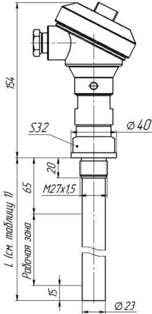
Рисунок Б.5 - ПП-064, ПП-064И, ПП-066, ПП-066И, ПП-083, ПП-083И, ПП-084, ПП-084И ПП-264, ПП-264И, ПП-266, ПП-266И, ПП-283, ПП-283И, ПП-284, ПП-284И
