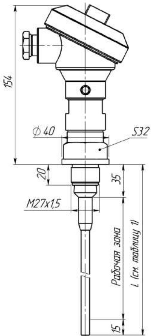
Рисунок Б.4 - ПП-025, ПП-025И, ПП-225, ПП-225И
