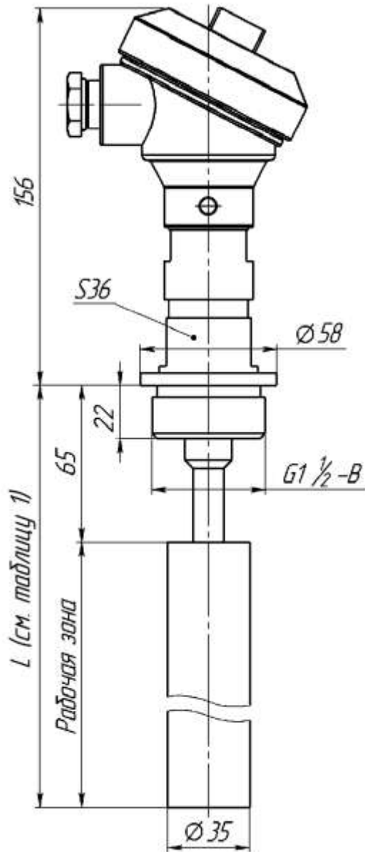
Рисунок Б.3 - ПП-016, ПП-016И, ПП-216, ПП-216И
