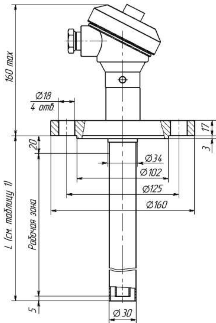
Рисунок Б.6 - ПП-082, ПП-082И, ПП-282, ПП-282И
