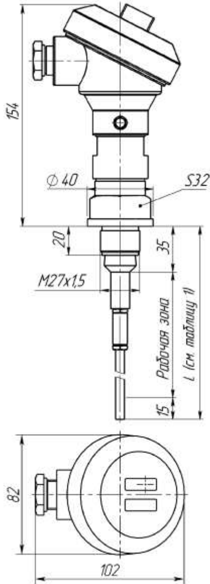
Рисунок Б.1 - ПП-005, ПП-005И, ПП-205, ПП-205И
